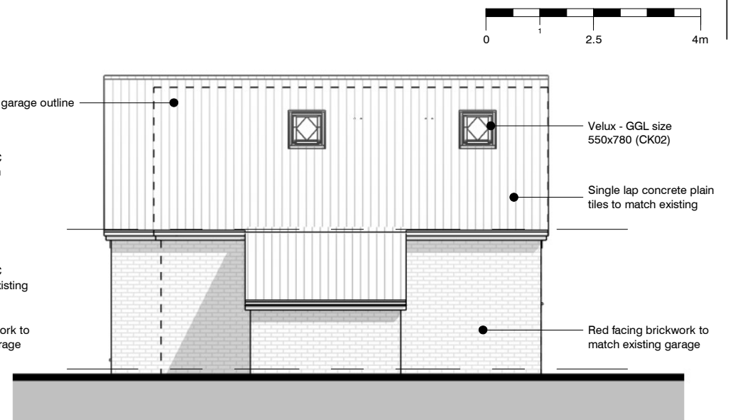
4 West Elevation 1 : 100 @A3
