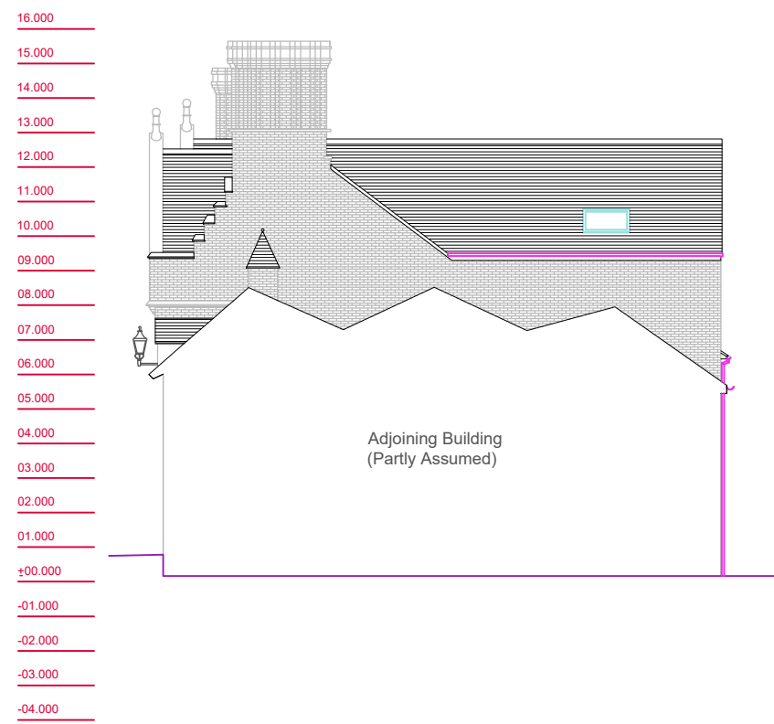
Right Elevation
