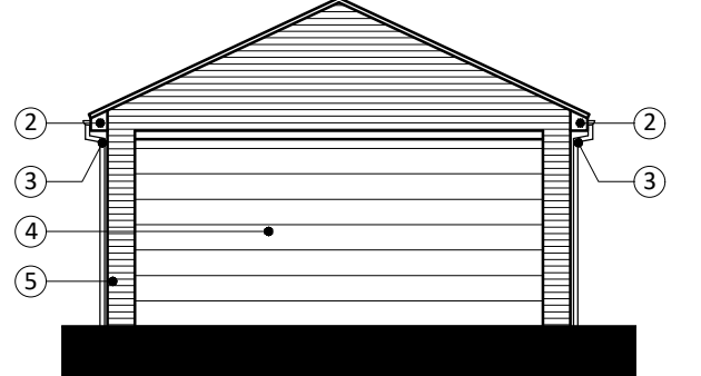
ELEVATION D-D
