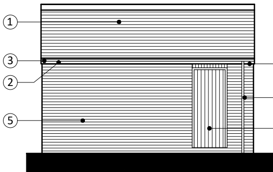
ELEVATION C-C
