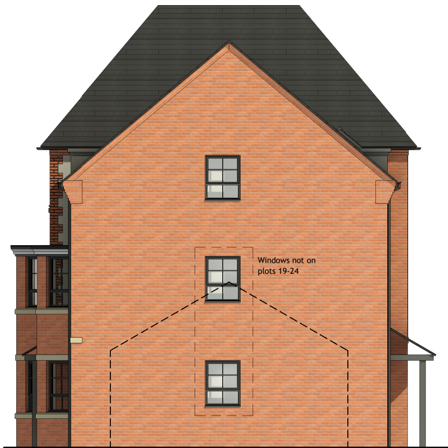
Right Elevation
