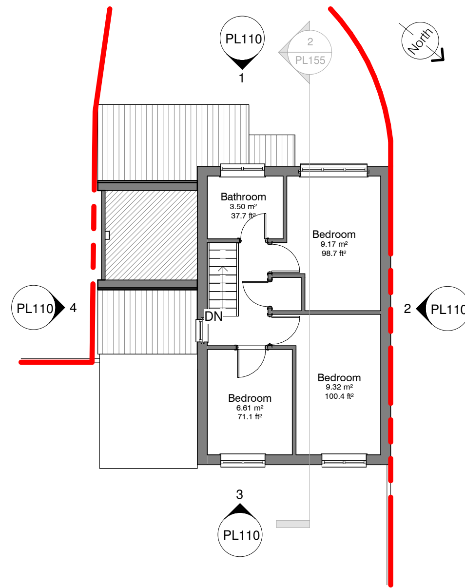
2 FIRST - Existing 1 : 100 @A3
