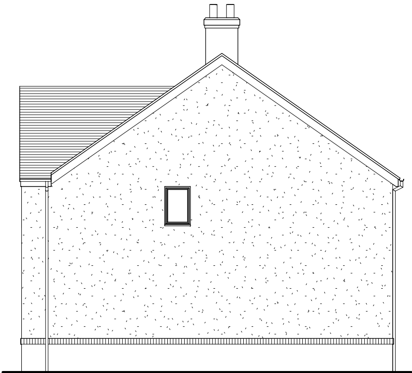
Right Elevation
