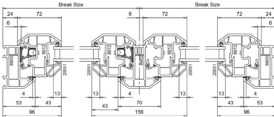
Section D-D
