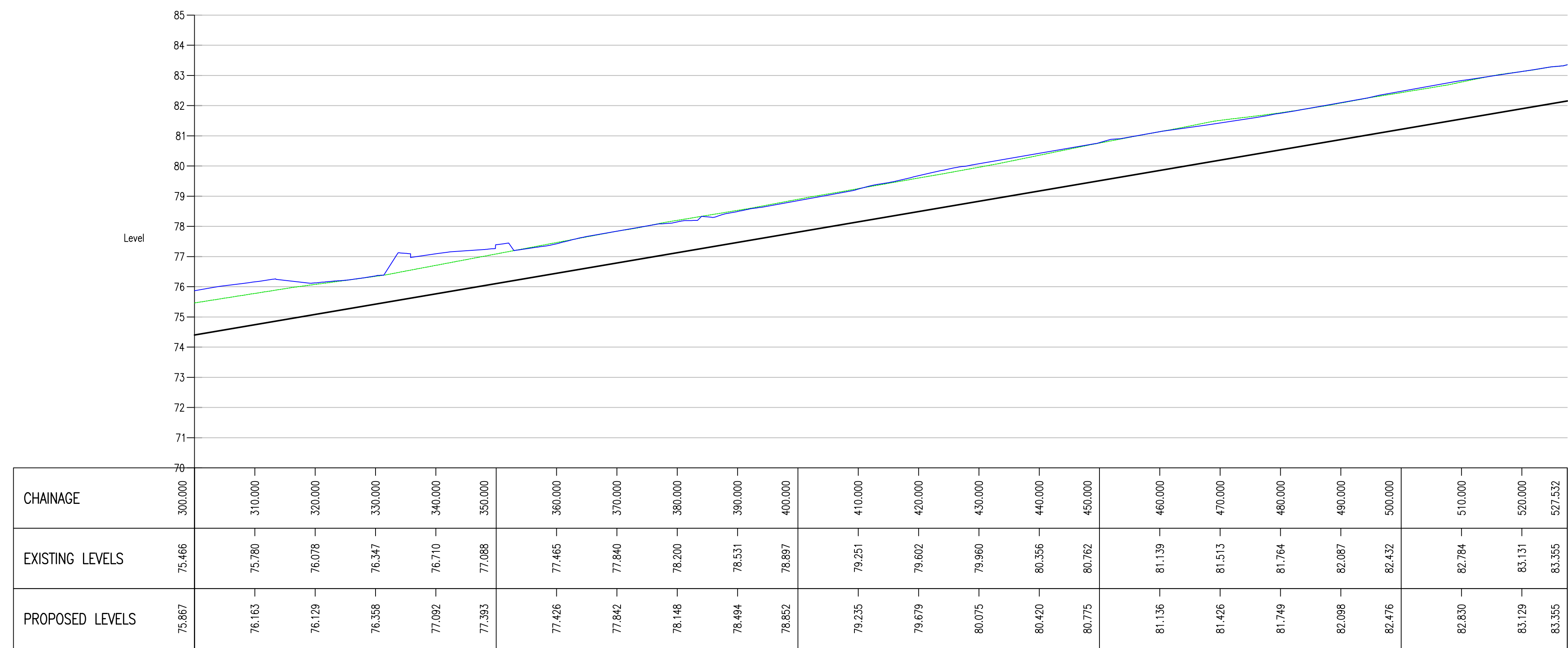
PR-RM CH 300.000m TO 527.532m SCALE: H 1:500,V 1:100. DATUM: 70.000
