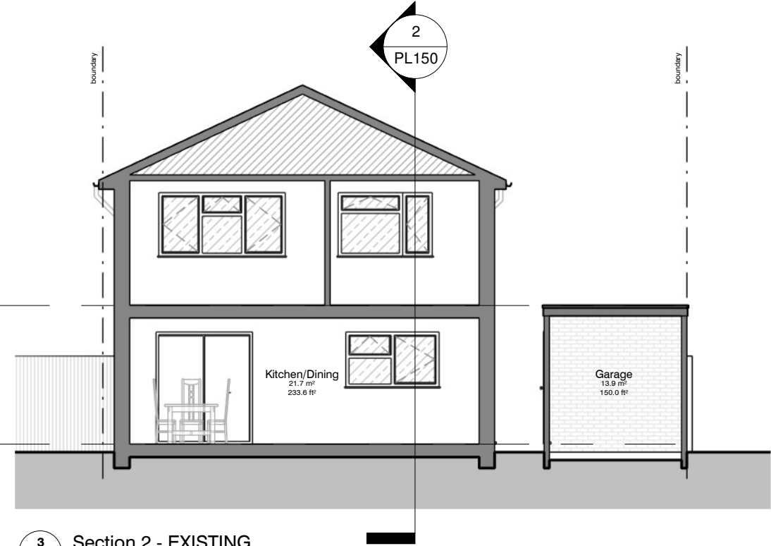
3 Section 2 - EXISTING 1 : 100 @A3
