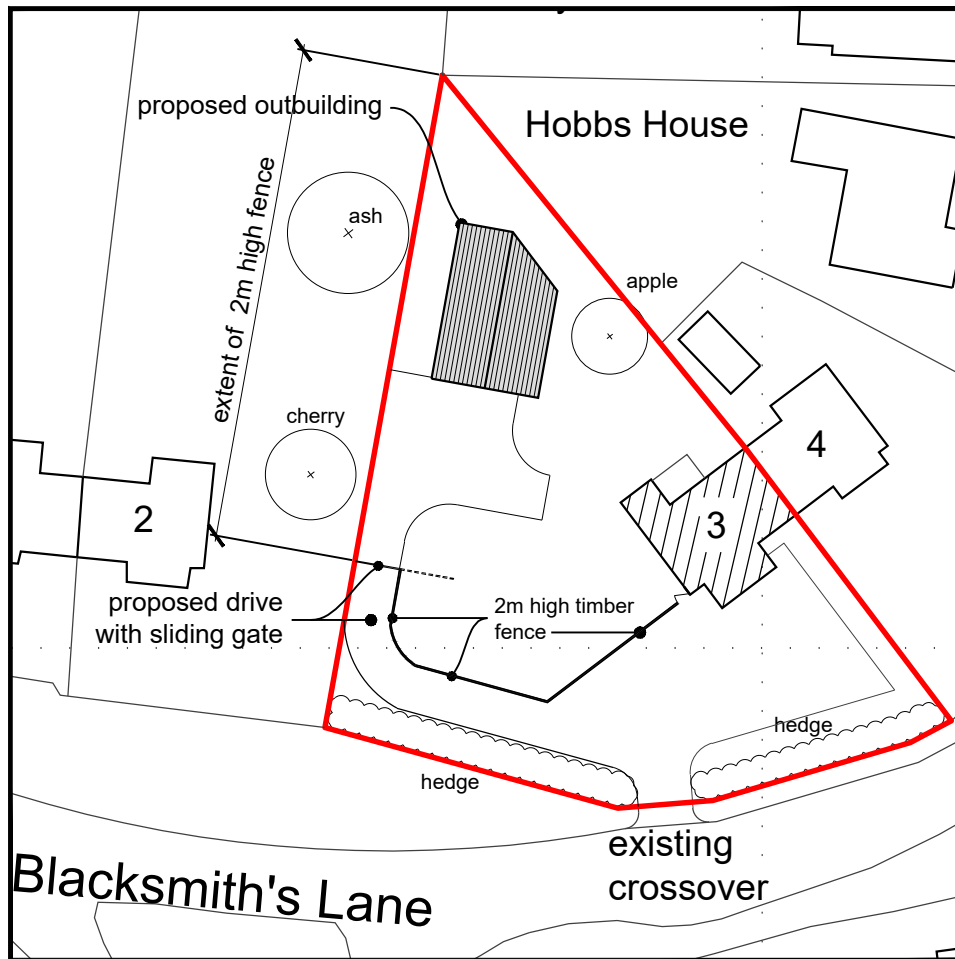
Site Plan 1:500
