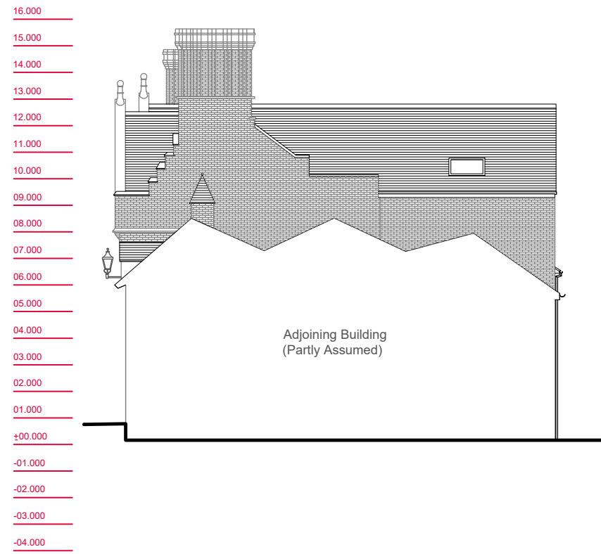
Right Elevation
