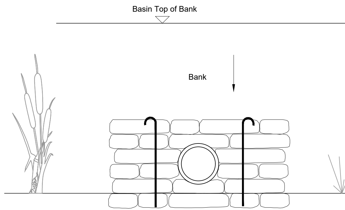
ELEVATION
