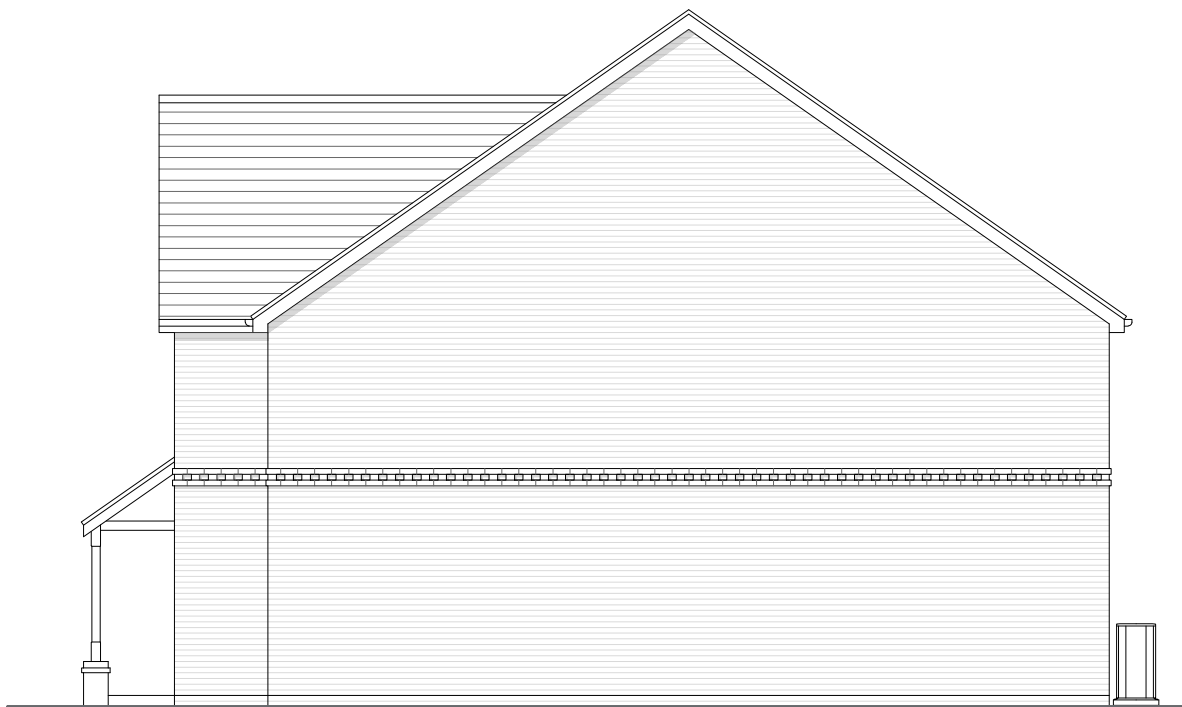
Elevation B
