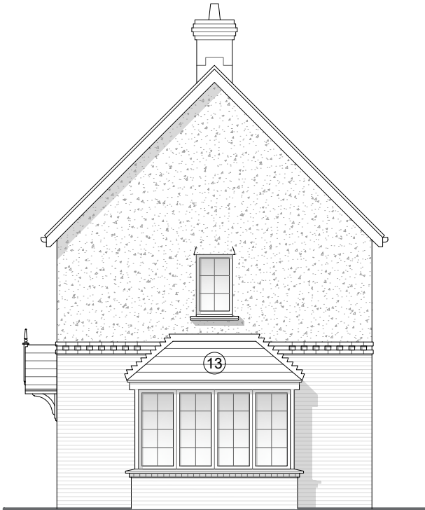
Elevation B
