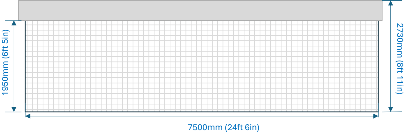
LH ELEVATION
