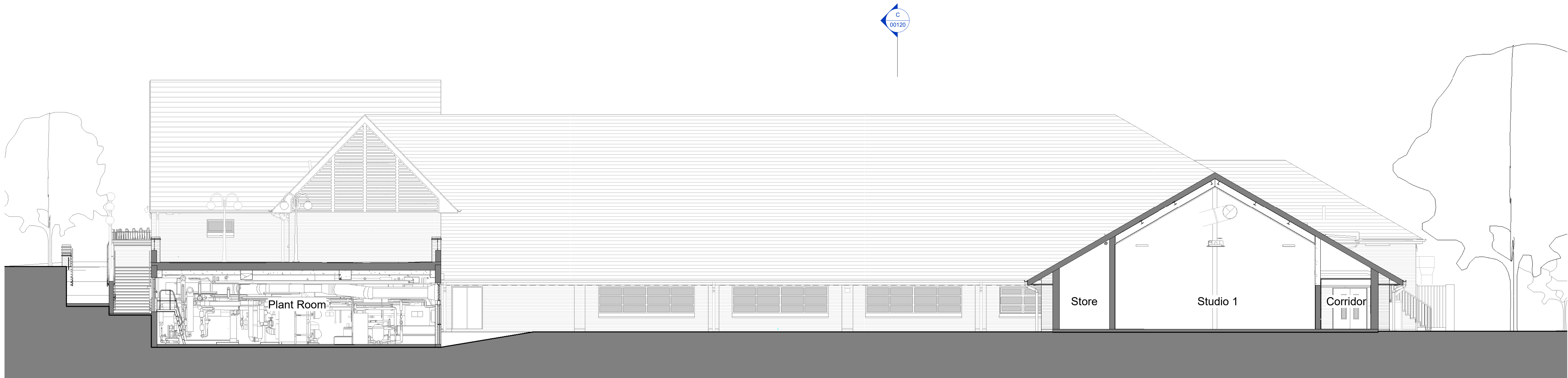
Section A 1 : 100
