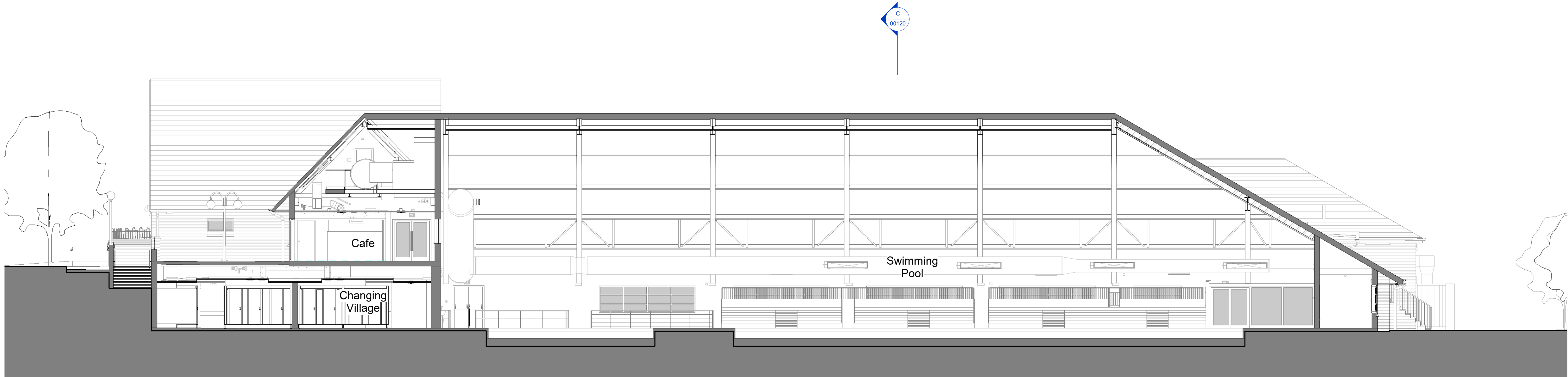
Section B 1 : 100
