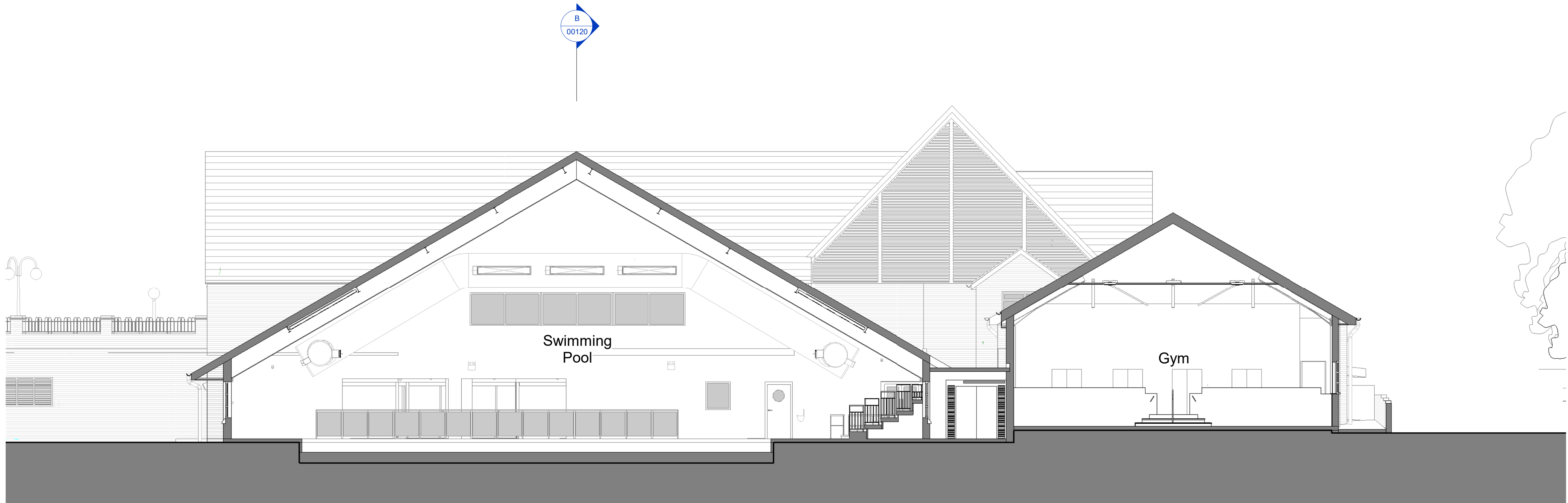
Section C 1 : 100
