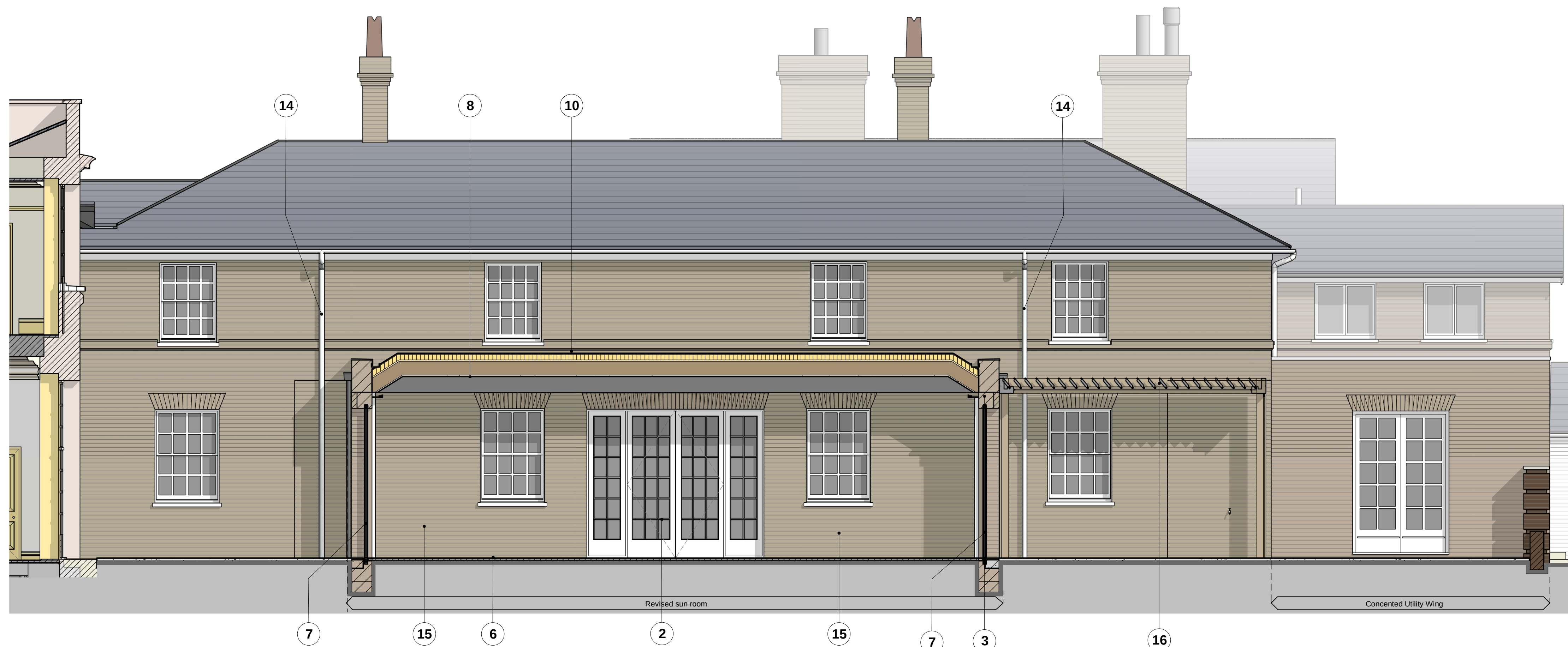
1 Sun Room - Section A 1 : 50
