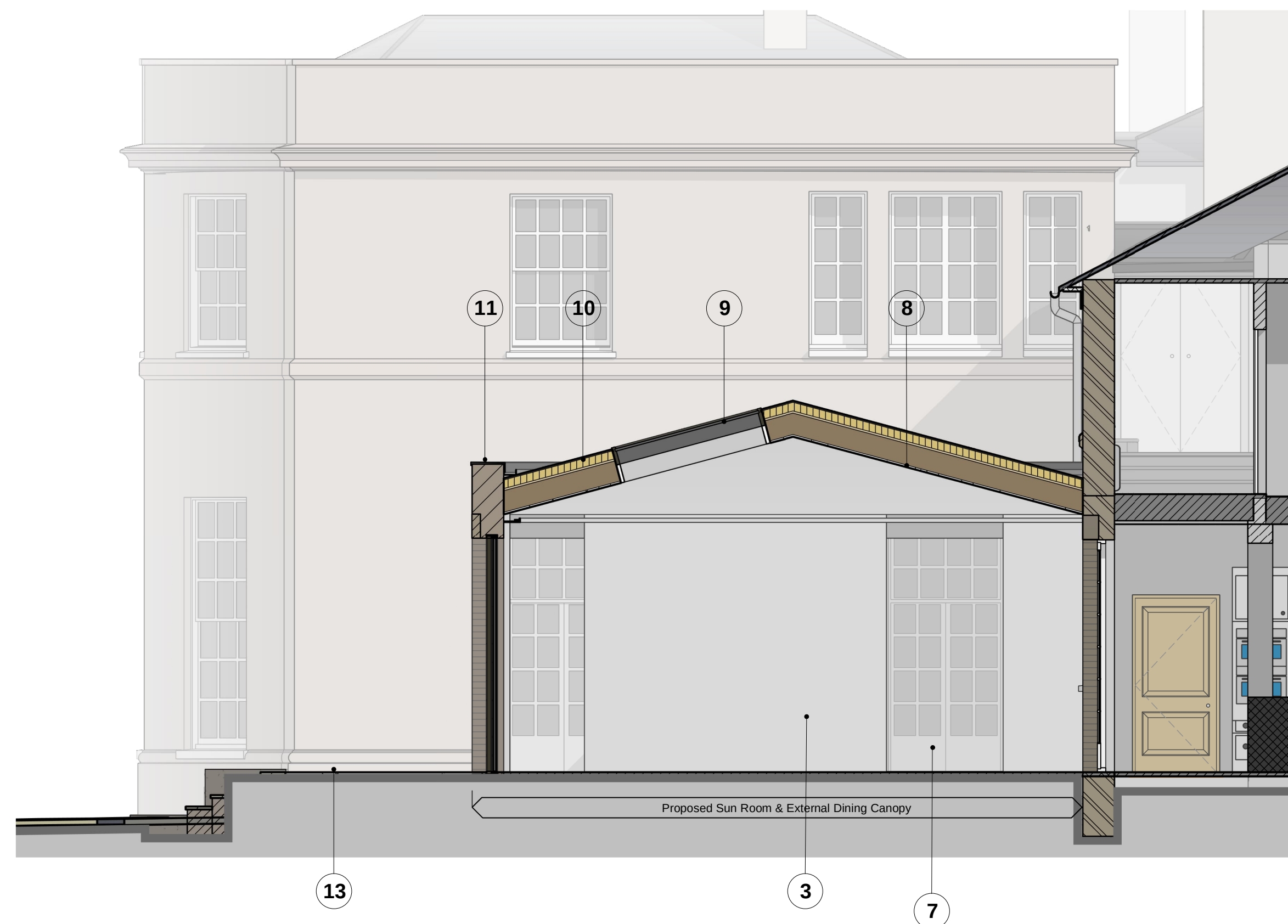
2 Sun Room - Section B 1 : 50
