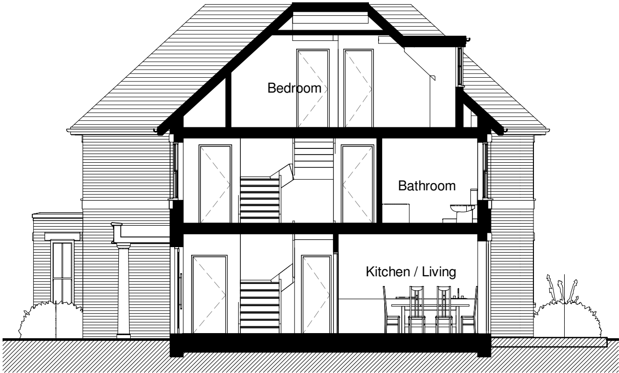
PLOT 2 Section B-B 1 : 100
