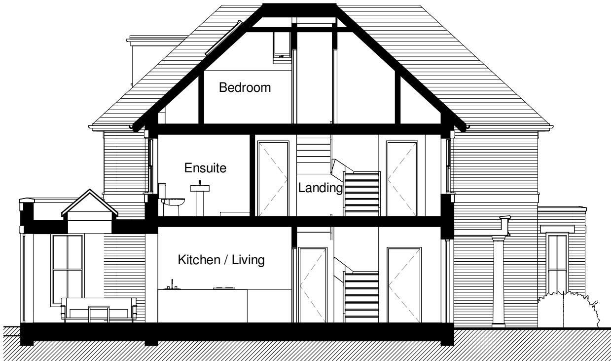
Section A-A 1 : 100
