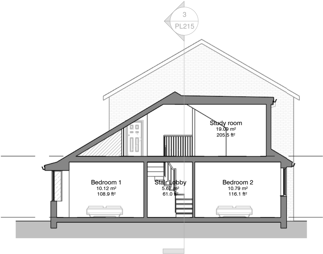
1 Section 1 1 : 100 @A3
