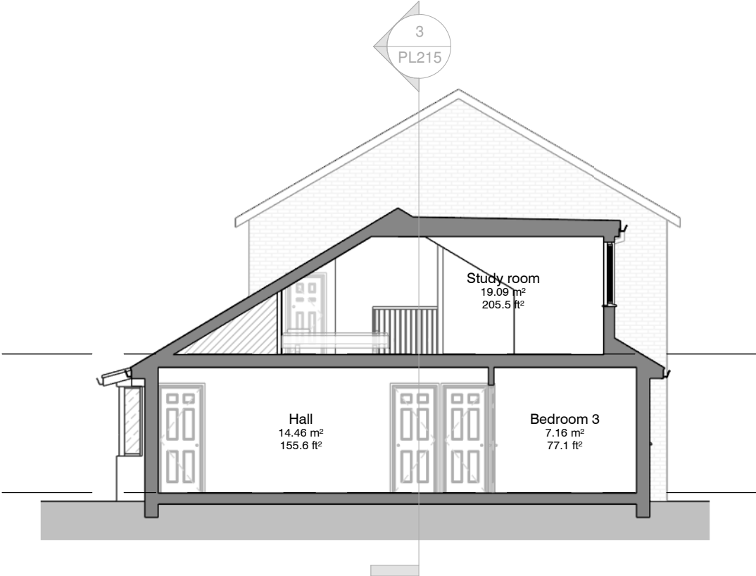
2 Section 2 1 : 100 @A3
