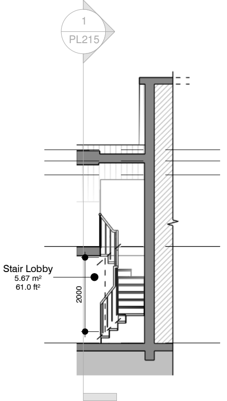
3 Section 3 1 : 100 @A3
