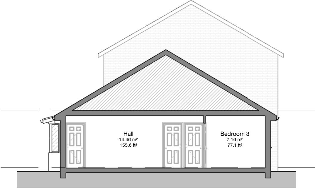
5 Section 2 - Existing 1 : 100 @A3
