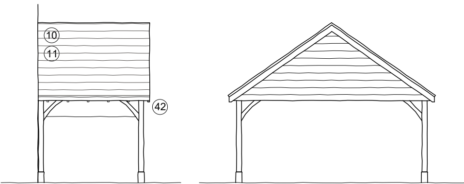
Elevation A Elevation B
