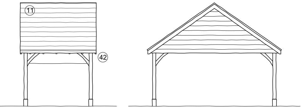
Elevation A Elevation B
