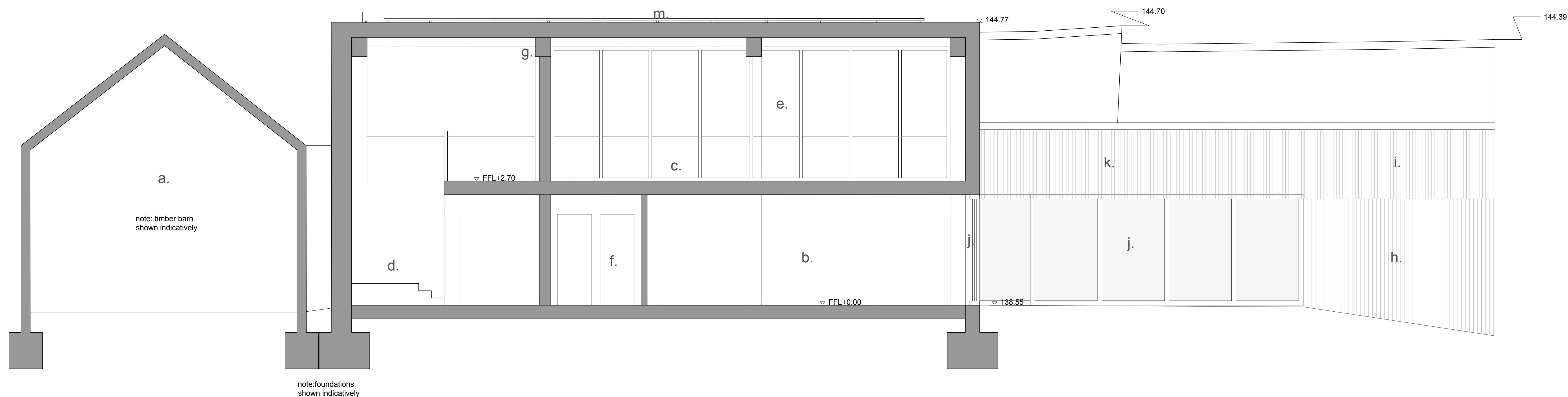
Section A-A'
