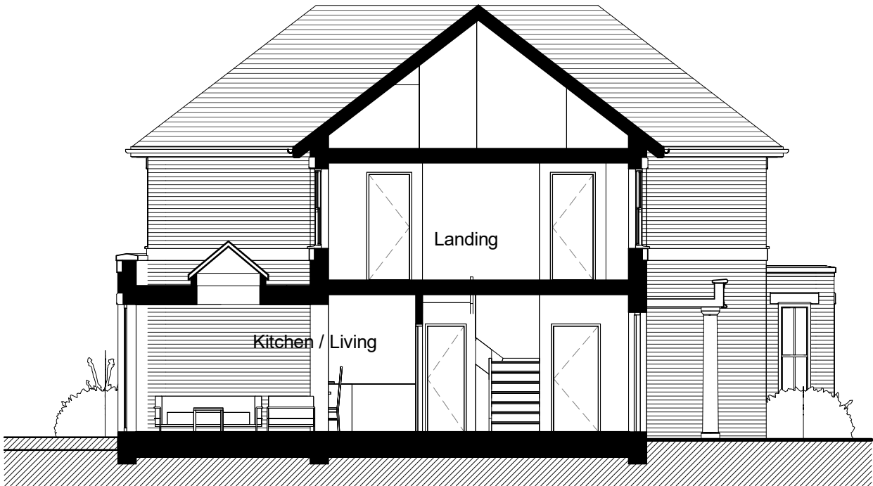
Section A-A 1 : 100
