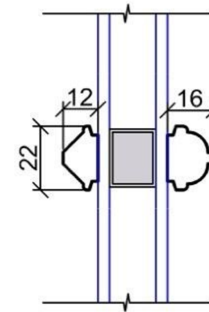
Glazing Bar
