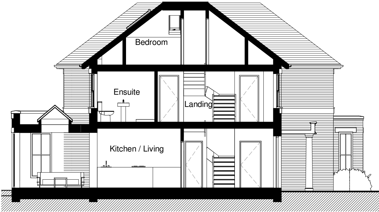
Section A-A 1 : 100
