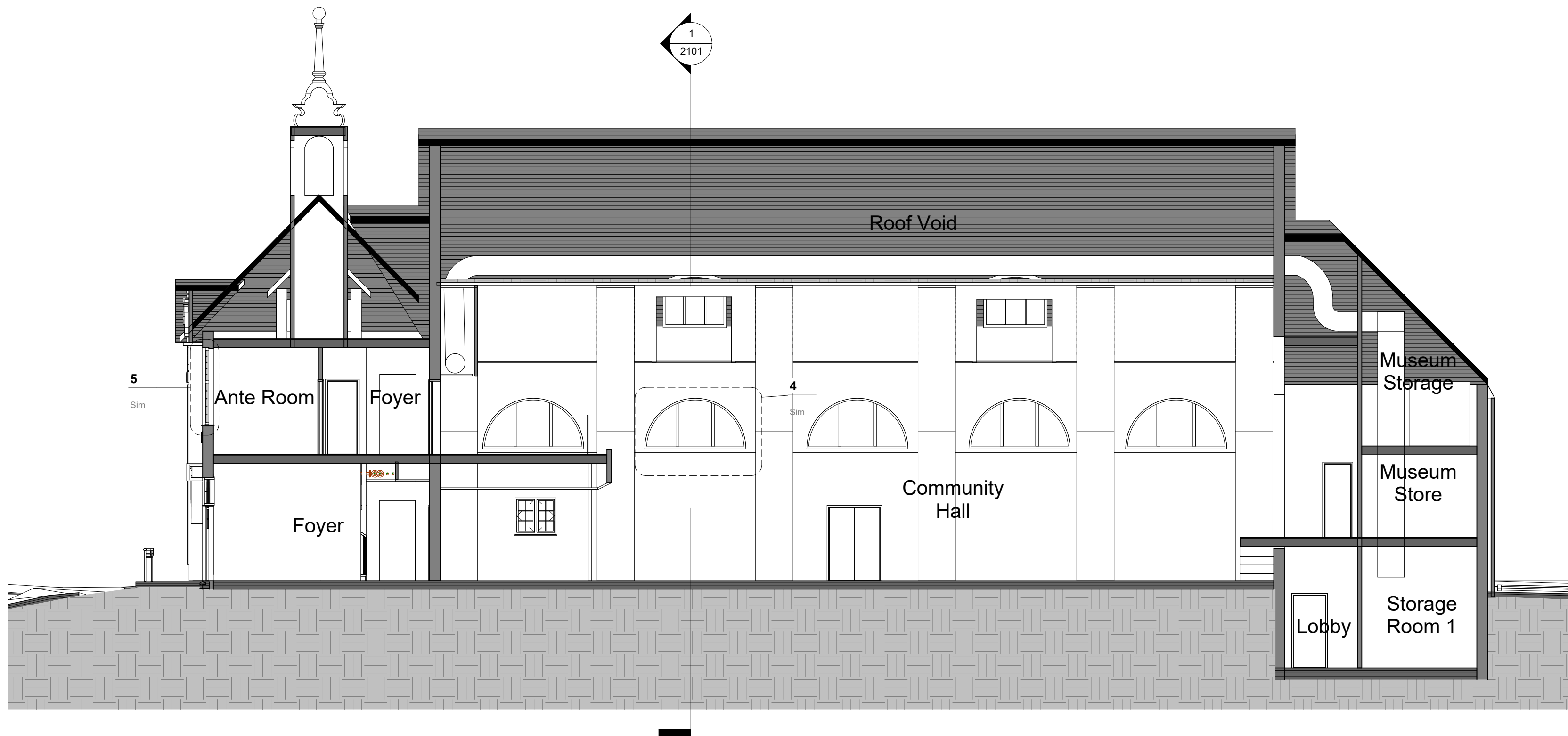
2 Existing - Long Section 1 : 100
