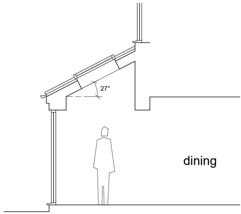
Section A-A 1:50
