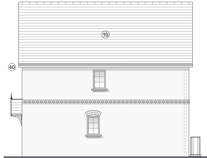
Elevation B
