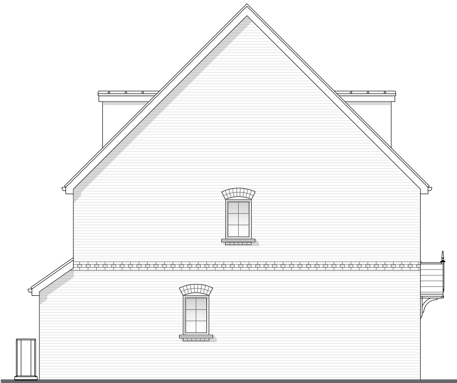
Elevation B
