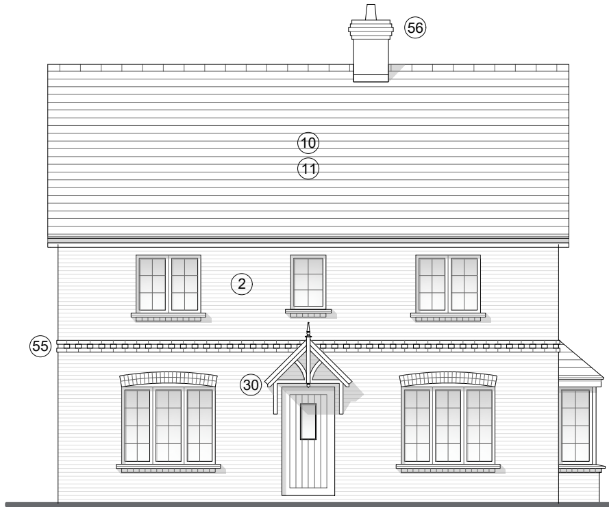
Elevation A
