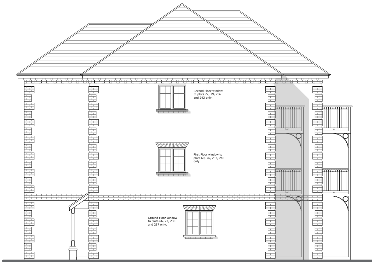
Elevation B
