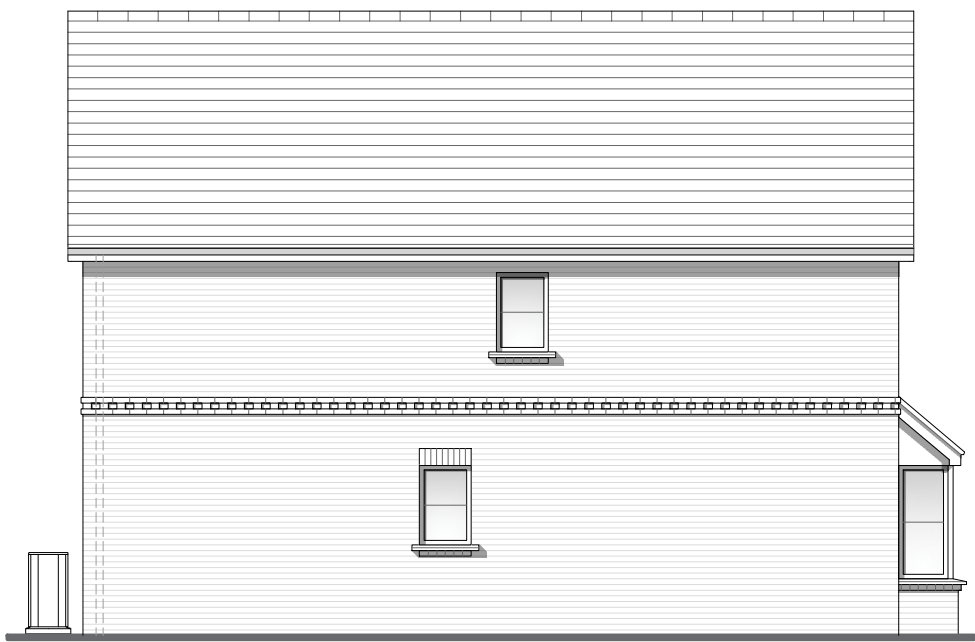
Elevation B
