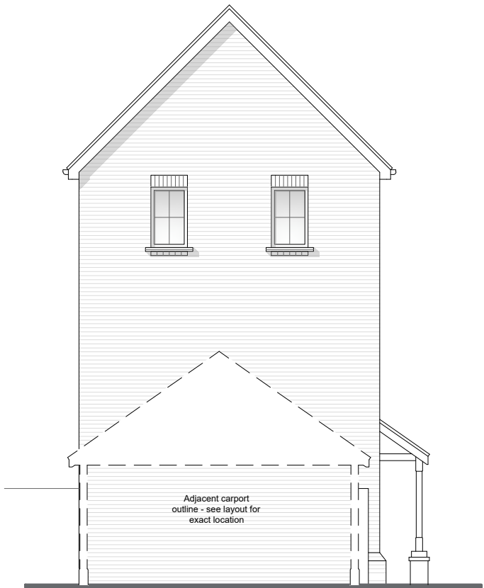
Elevation B
