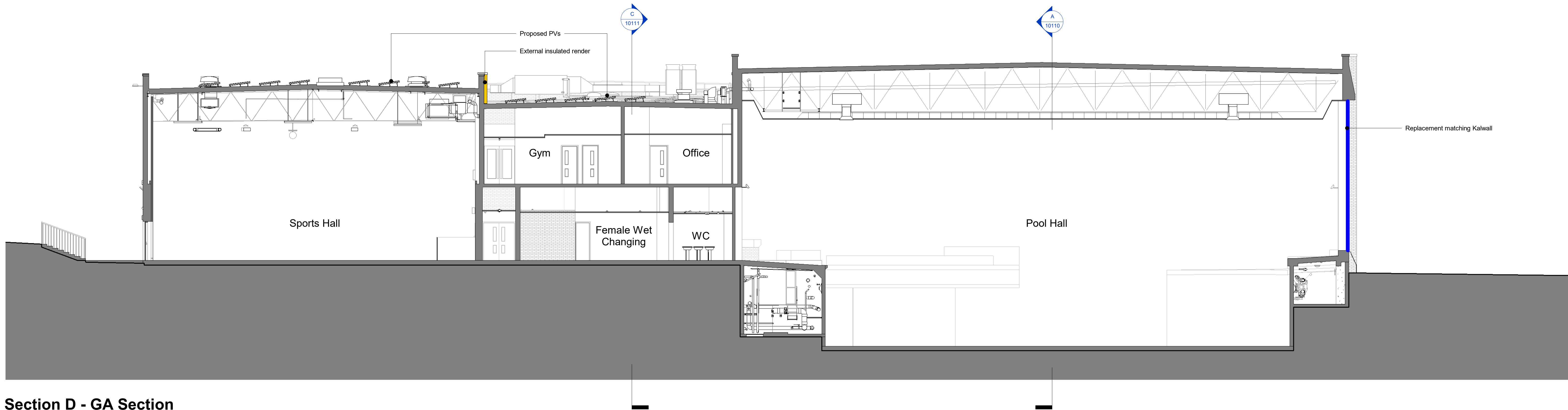
Section D - GA Section 1 : 100
