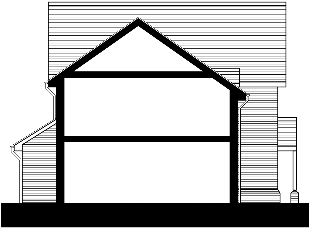
SIDE ELEVATION (A-A)
