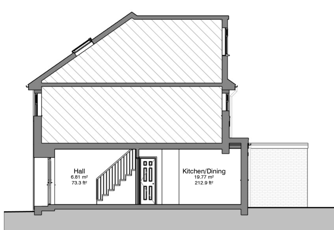
4 Section 1 - Existing 1 : 100 @A3
