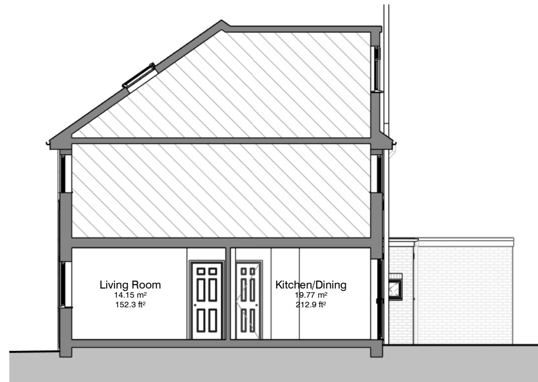
5 Section 2 - Existing 1 : 100 @A3
