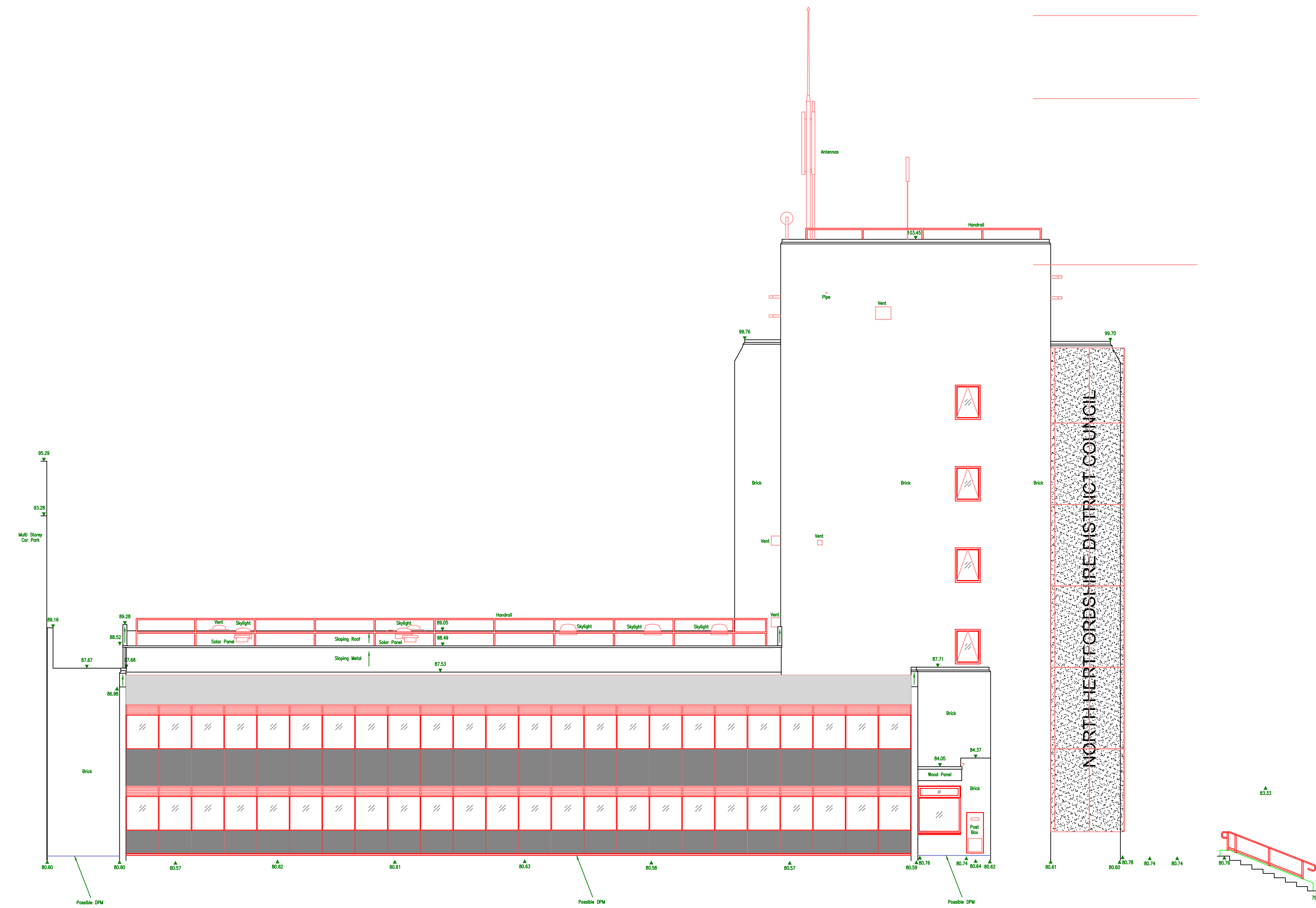
Elevation 2
