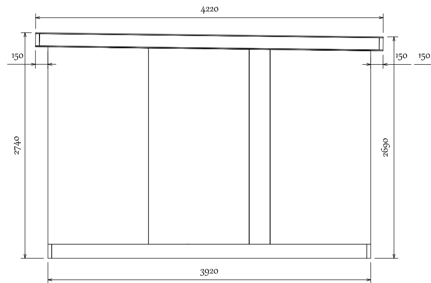
Bottom
