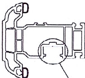
EUROGROOVE
