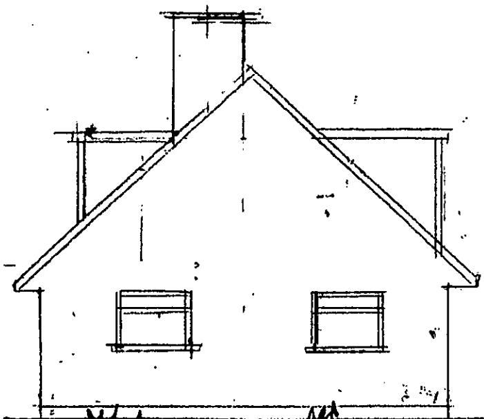
end elevation
