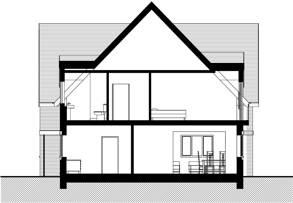
Section BB 1 : 100
