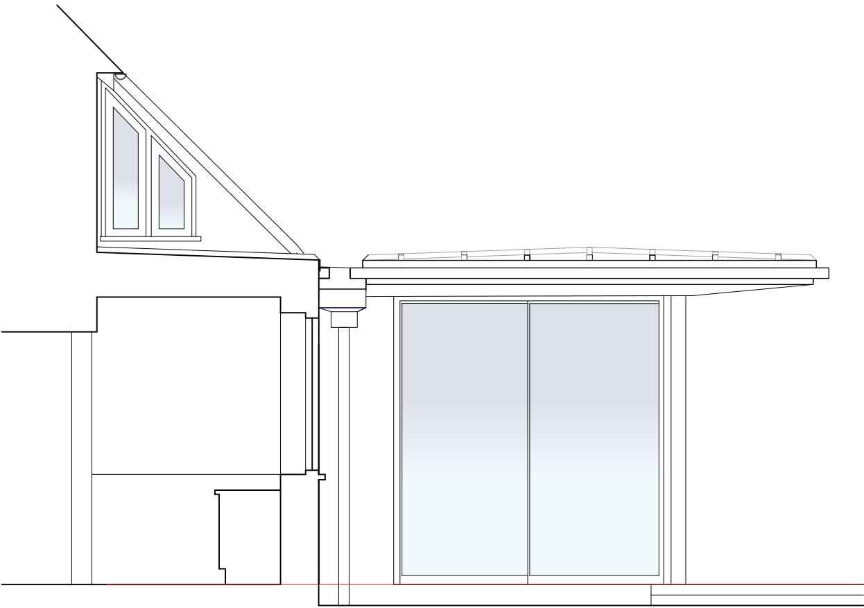
SECTION D-D
