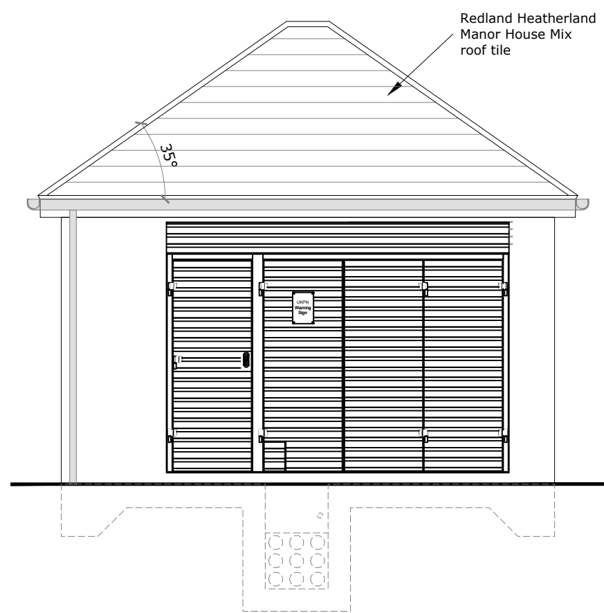
Elevation A
