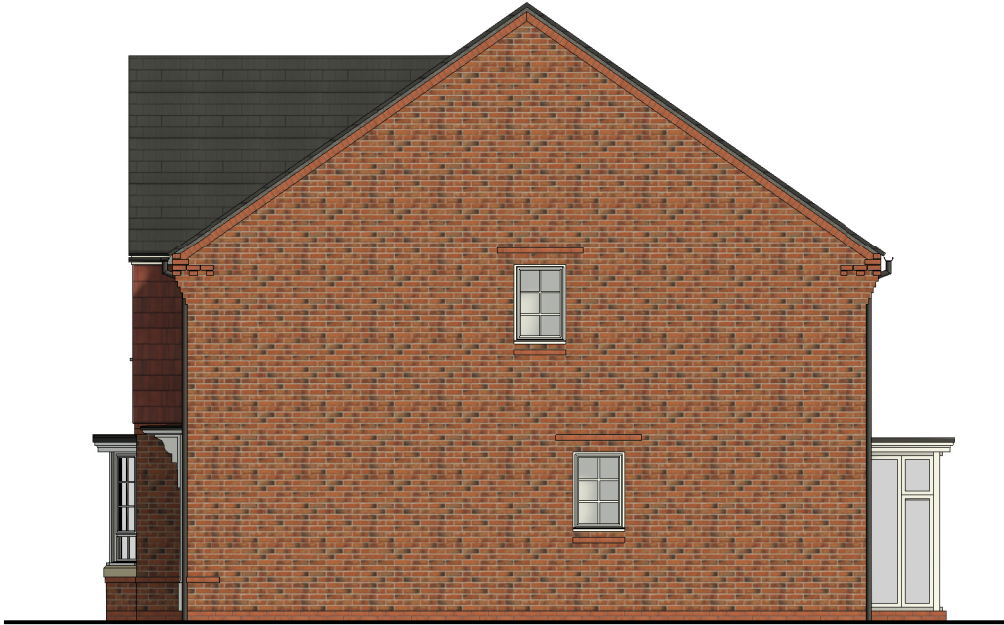
Right Elevation
