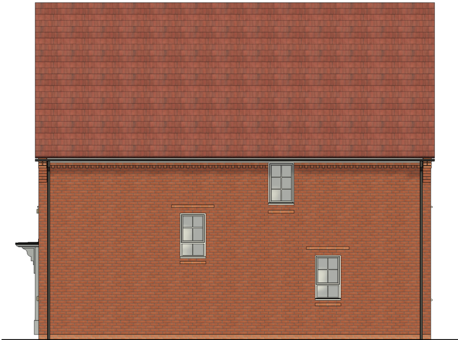
Right Elevation
