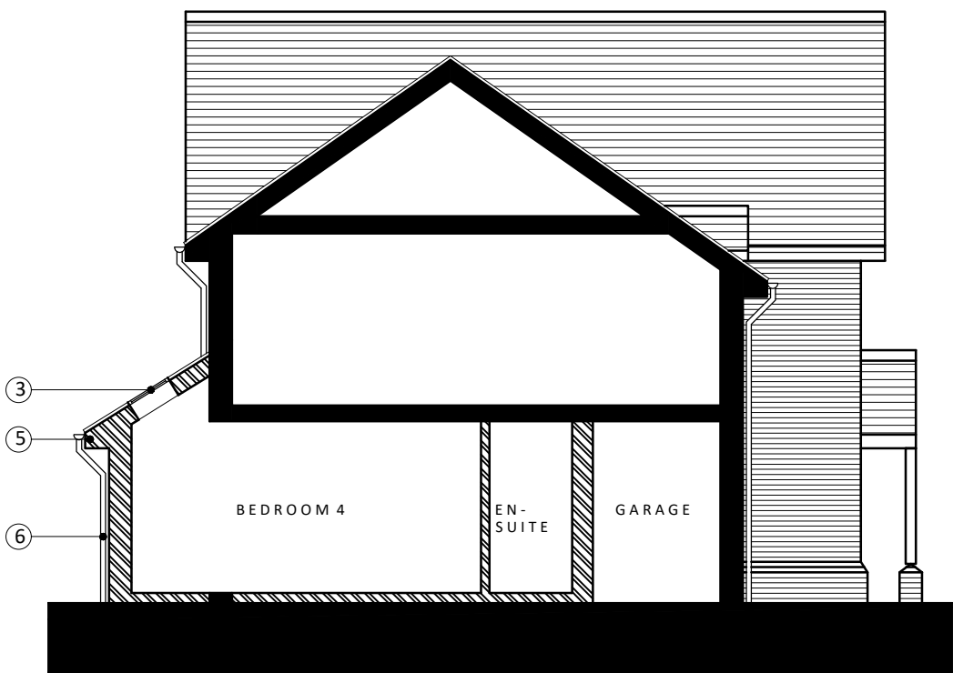
SIDE ELEVATION (A-A)
