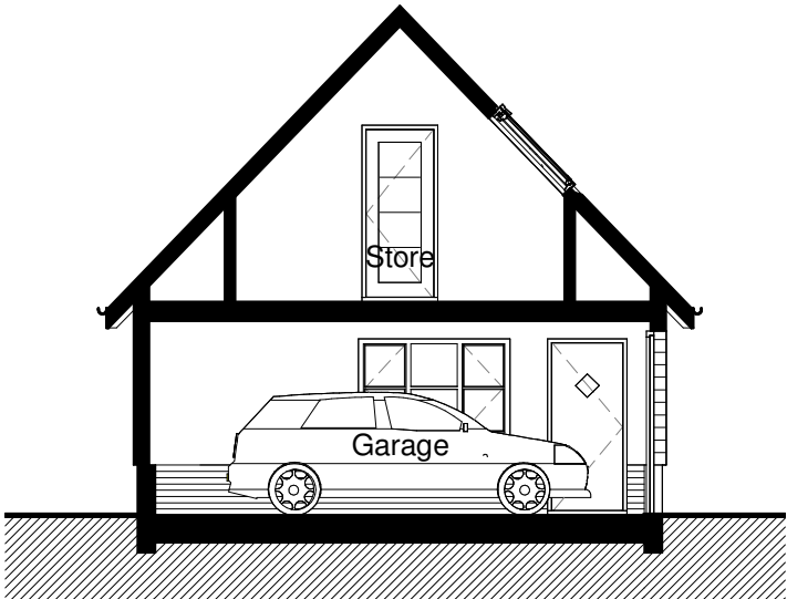
Section A-A 1 : 100
