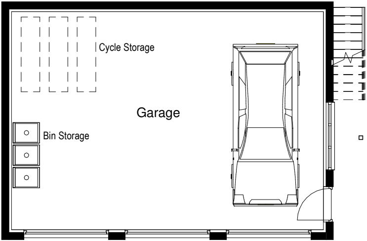
Garage Floor Plan 1 : 100
