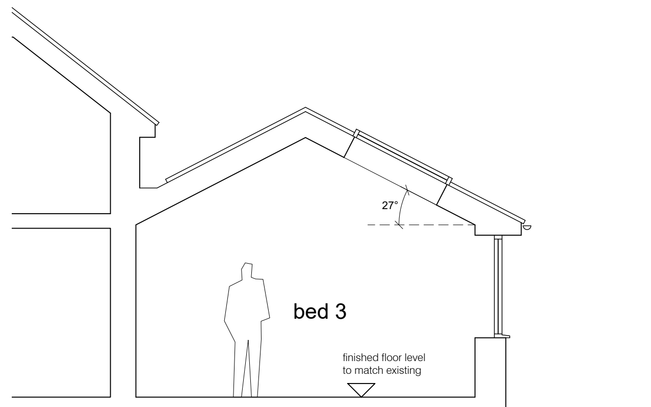
Section A-A 1:50
