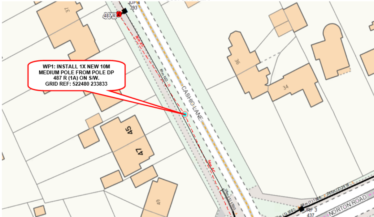
-DUCT DIAGRAM-2-
