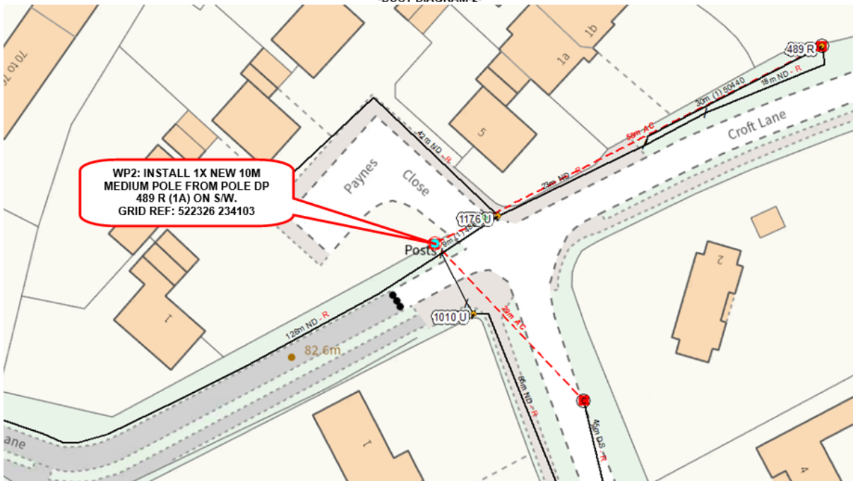
-DUCT DIAGRAM-2-
