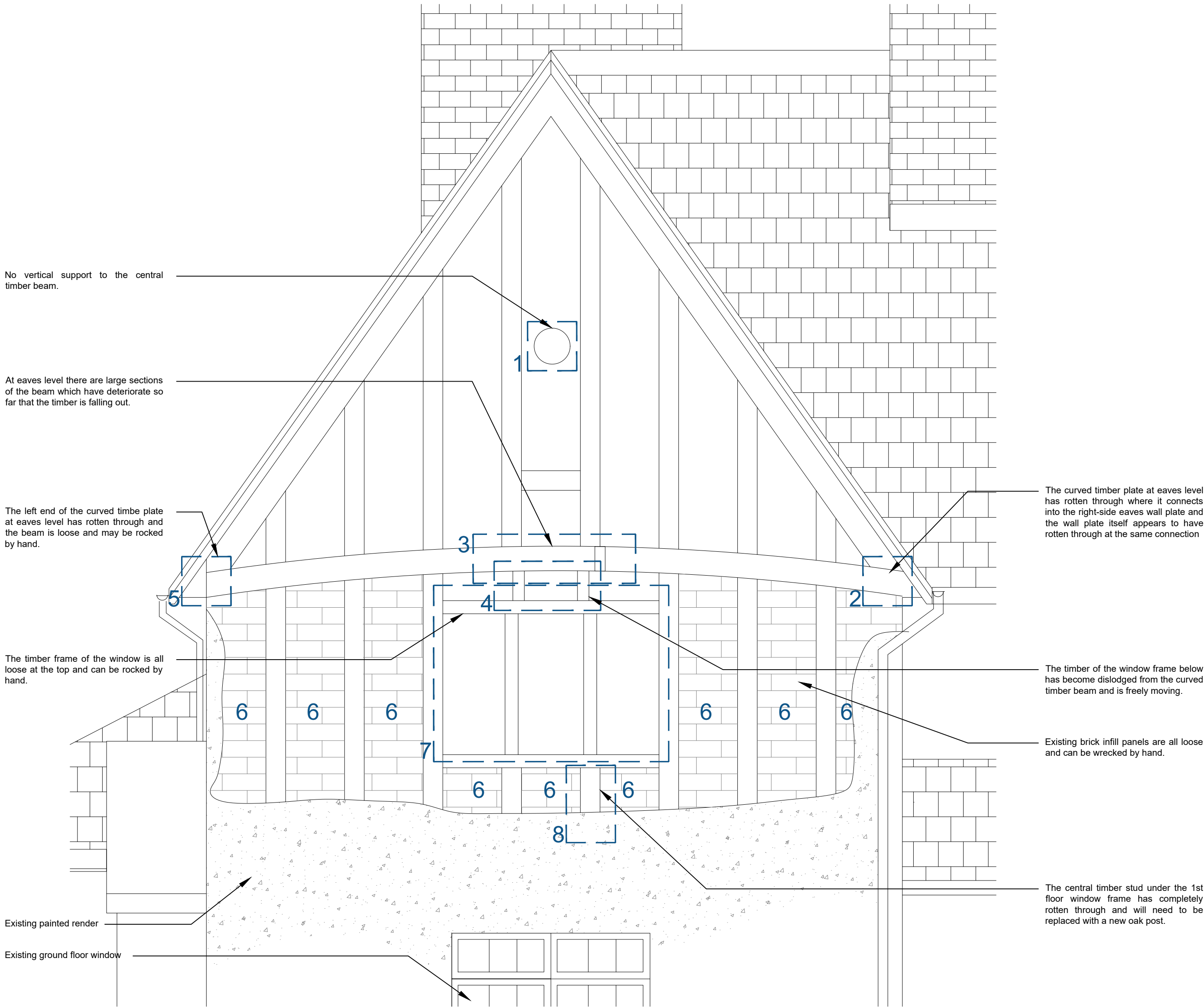
2 Existing Gable Scale: 1:20
